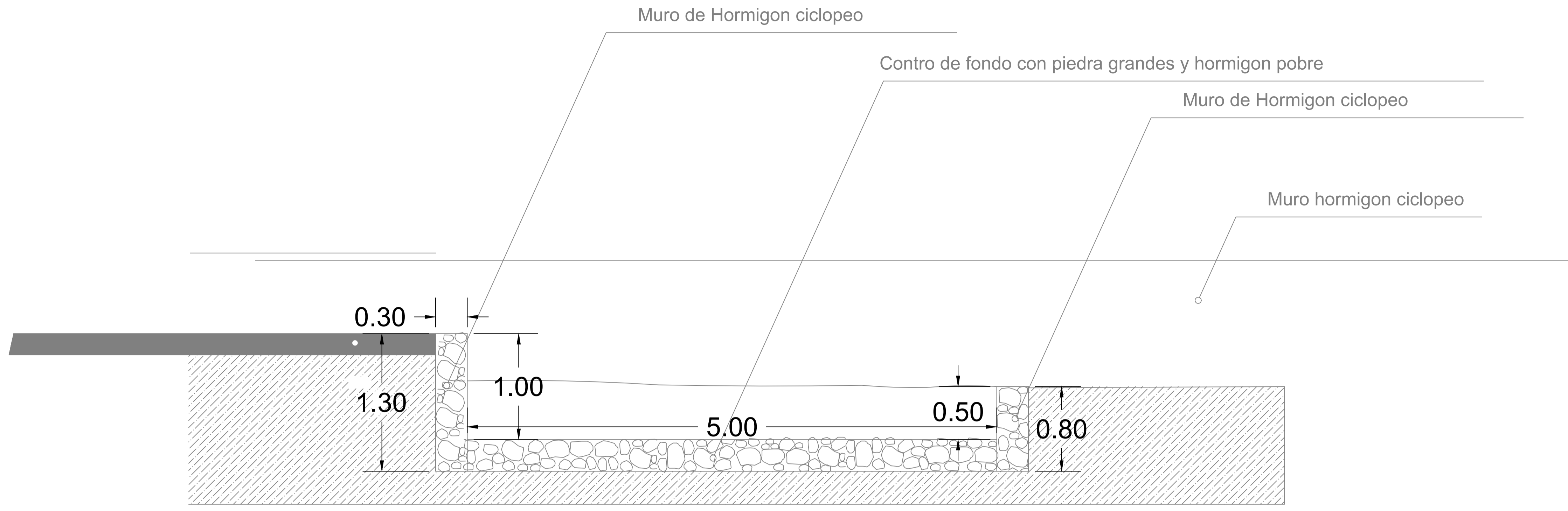
CORTE LONGITUDINAL
