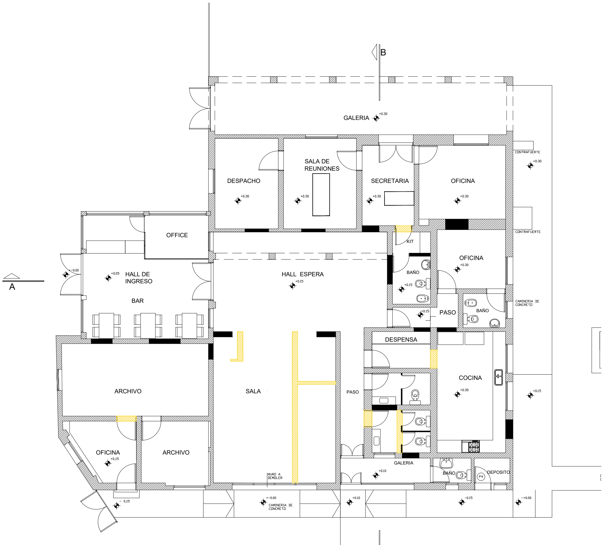
PLANTA MUROS A DEMOLER Y A EJECUTAR
