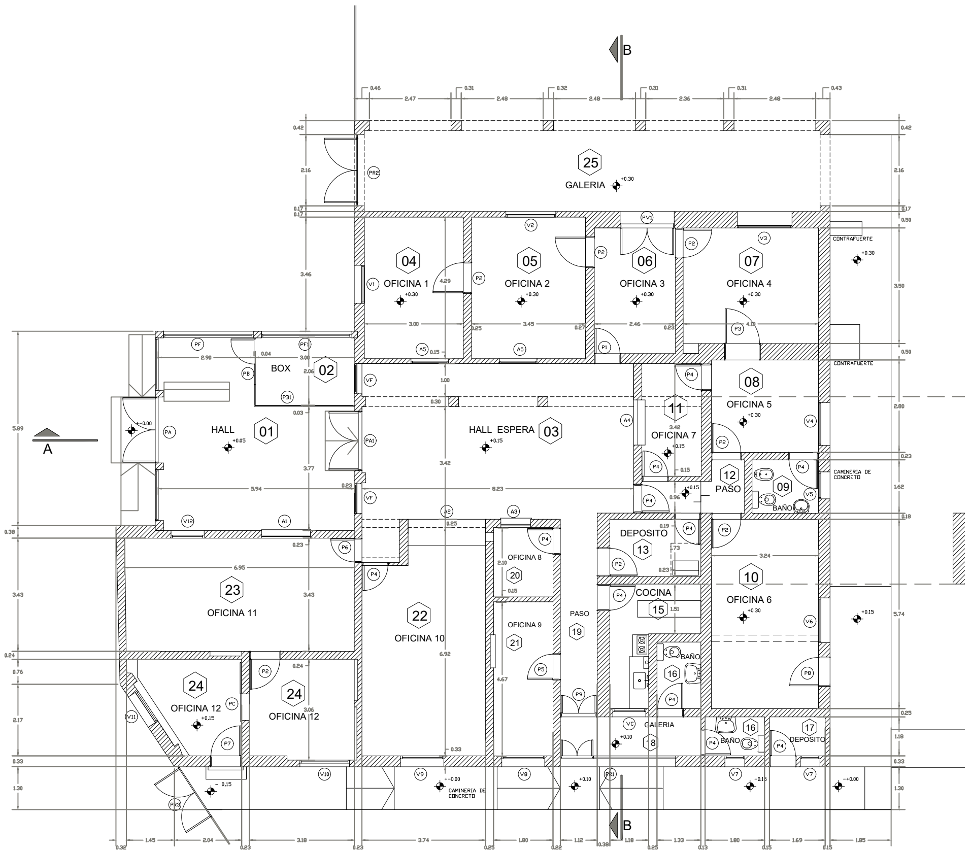
PLANO DE PLANTA ORIGINAL EXISTENTE
