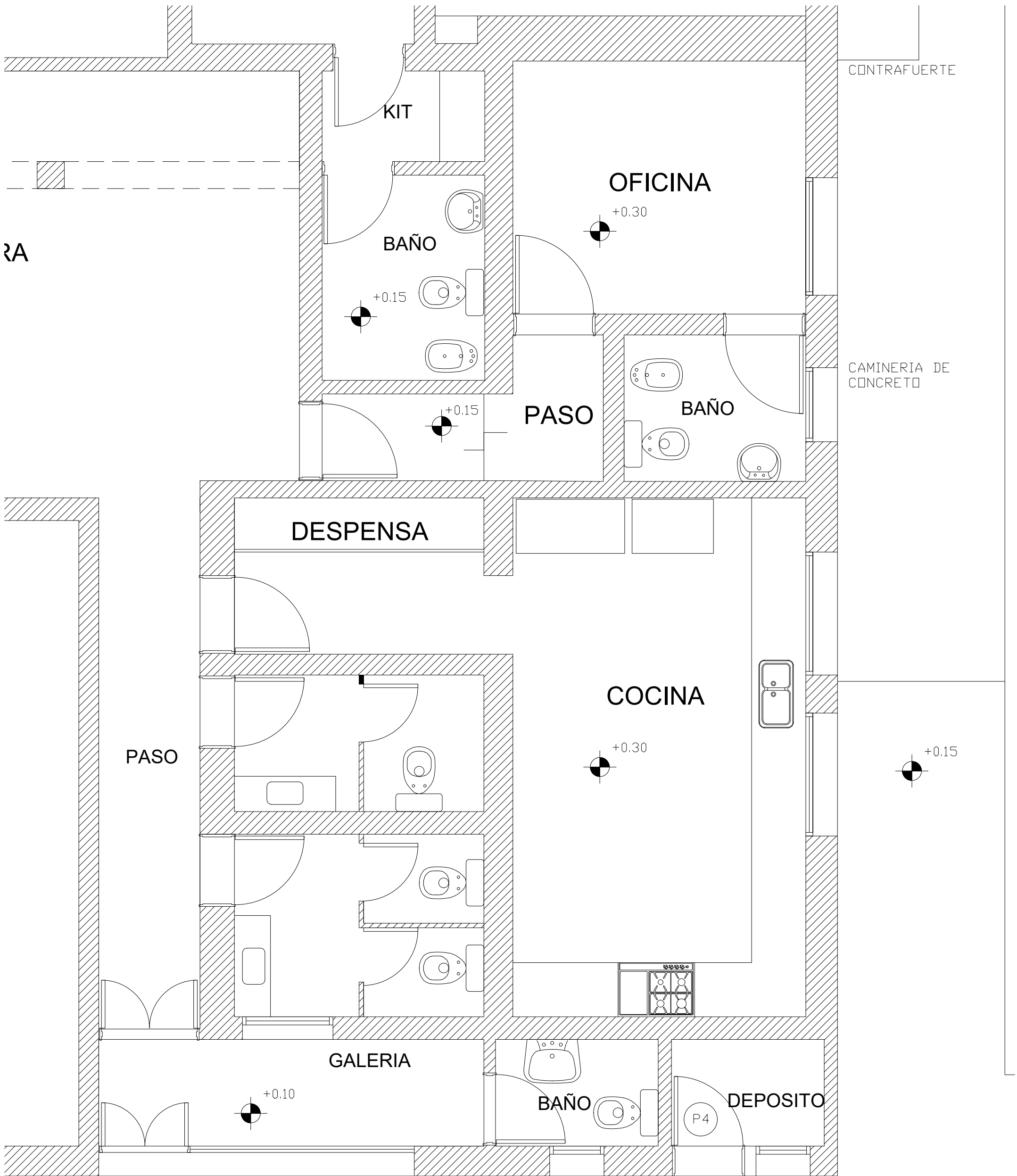
PLANTA DETALLES SECTOR BAÑOS NUEVOS Y COCINA
